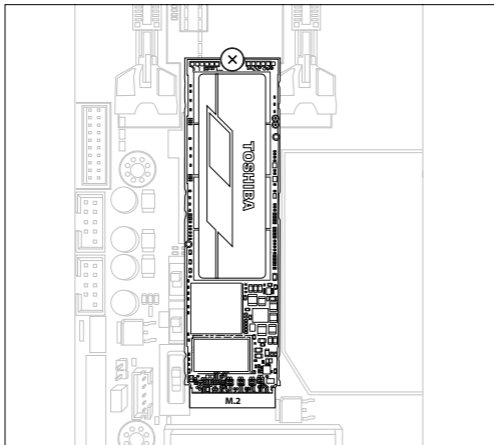
Image 3: Fixez le SSD NVMe de Toshiba avec la vis dans l'entretoise de la carte mère. Assurez-vous que le SSD est bien fixé.
