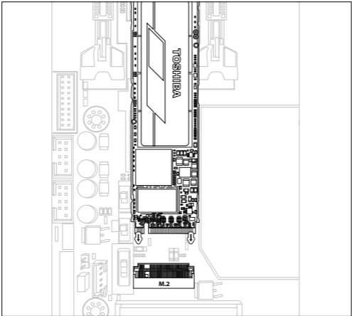
그림 2: Toshiba NVMe SSD를 M.2 슬롯에 삽입합니다.
